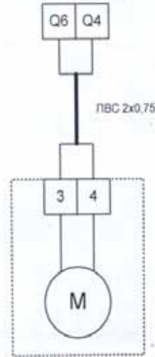
Сервопривод воздушной заслонки 230 вольта с возвратной пружиной
