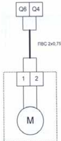
Сервопривод воздушной заслонки 24 вольта с возвратной пружиной
