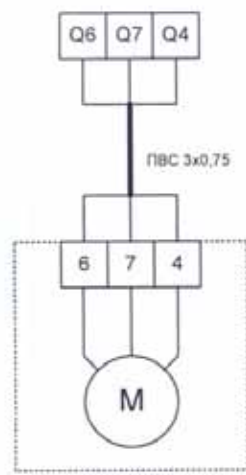
Сервопривод воздушной заслонки 230 вольт трехфазный
